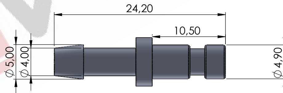
Conector aéreo gas macho mini E 4
