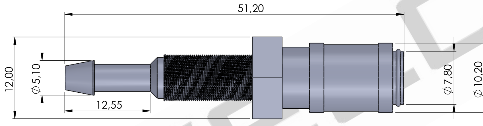
Conector chasis refrigeración hembra gas mini E 4
