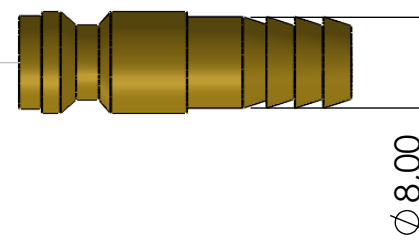
Conector aéreo refrigeración-gas macho E 8
