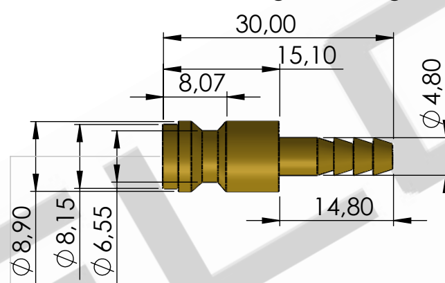
Conector aéreo refrigeración-gas macho E 6
