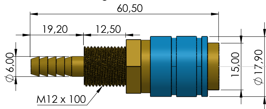
Conector chasis refrigeración hembra rojo E 6
