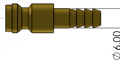
Conector aéreo refrigeración-gas macho E 8
