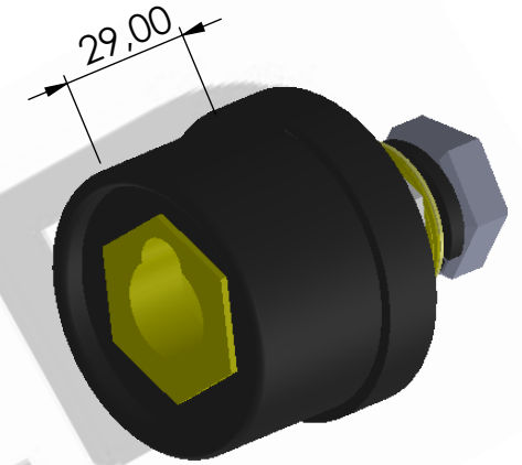
Conector chasis hembra 35-50 ST 13mm Carcasa 40mm
