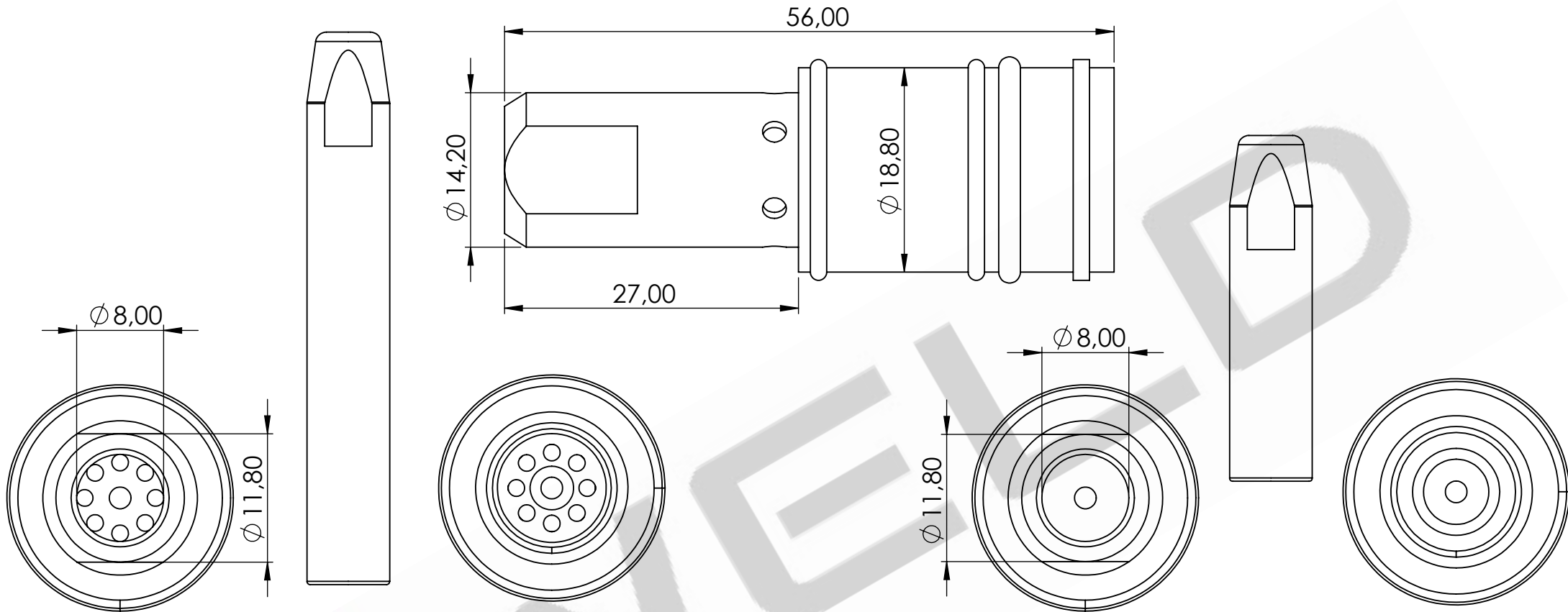
Portatubo Difusor BN 400(Puntas Largas)
